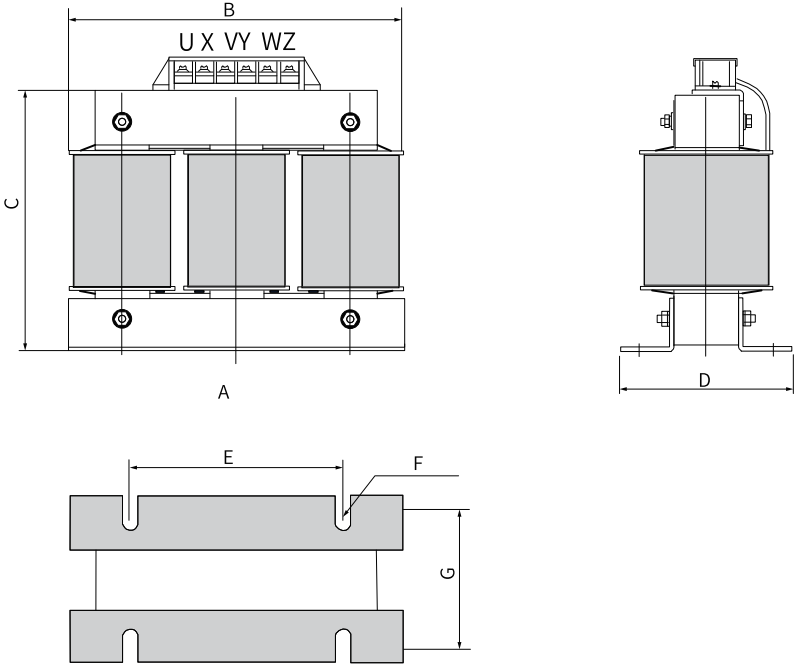
图7-11 20A交流输出电抗器尺寸图
