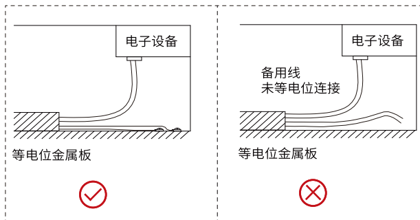
图9-11 多芯电缆有芯线剩余时的处理方法示意图
