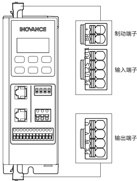
图9-18 T1~T2机型主回路端子分布图
