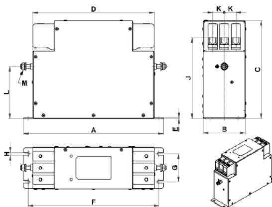
图7-13 FN 3287系列滤波器尺寸图（单位：mm）
