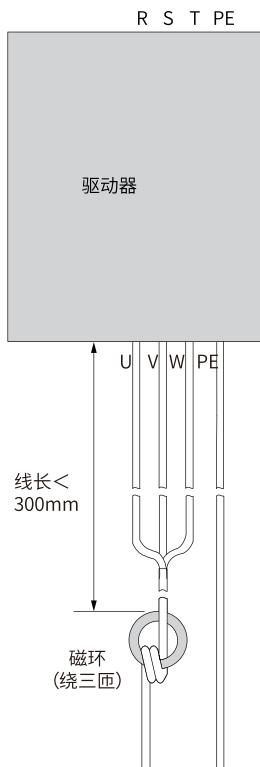
图9-2 磁环安装示意图
