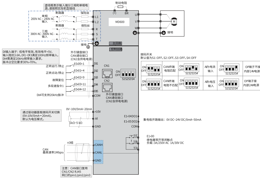
图9-17 三相/单相电源输入（MD600A-4T1R6~ MD600A-4T9R5B，MD600A-2S2R8~ MD600A-2S010B）端子接线图
