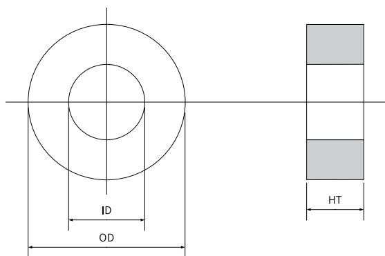
图7-14 磁环尺寸图
