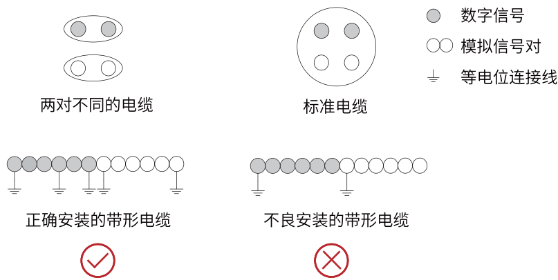
图9-9 不同类型信号电缆布线示意图
