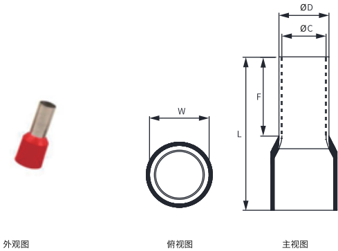
图7-5 管型预绝缘线耳（TG-JT型）外形及尺寸图
