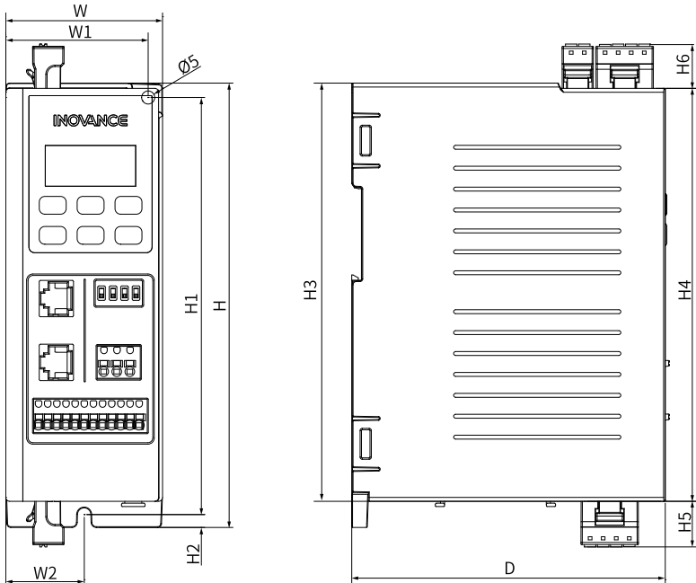
图8-4 T1~T2外型尺寸及安装尺寸示意图
