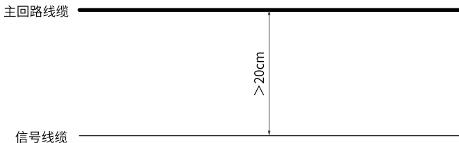
图9-7 线缆布线图
