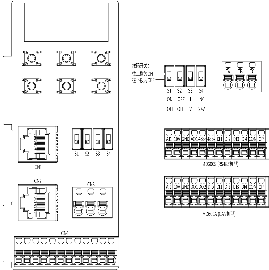
图9-21 控制回路端子分布图
