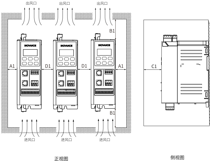
图8-2 安装空间示意图（并排安装）
