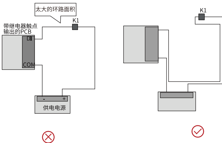
图9-12 避免布线环路过大示意图
