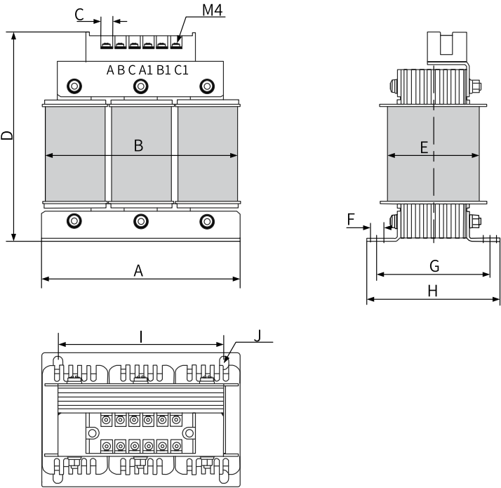
图7-7 10A-15A交流输入电抗器尺寸图
