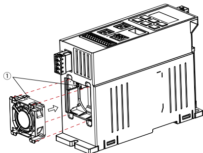
图8-7 风扇安装示意图
