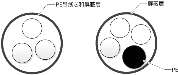
图7-3 推荐的动力线缆类型
