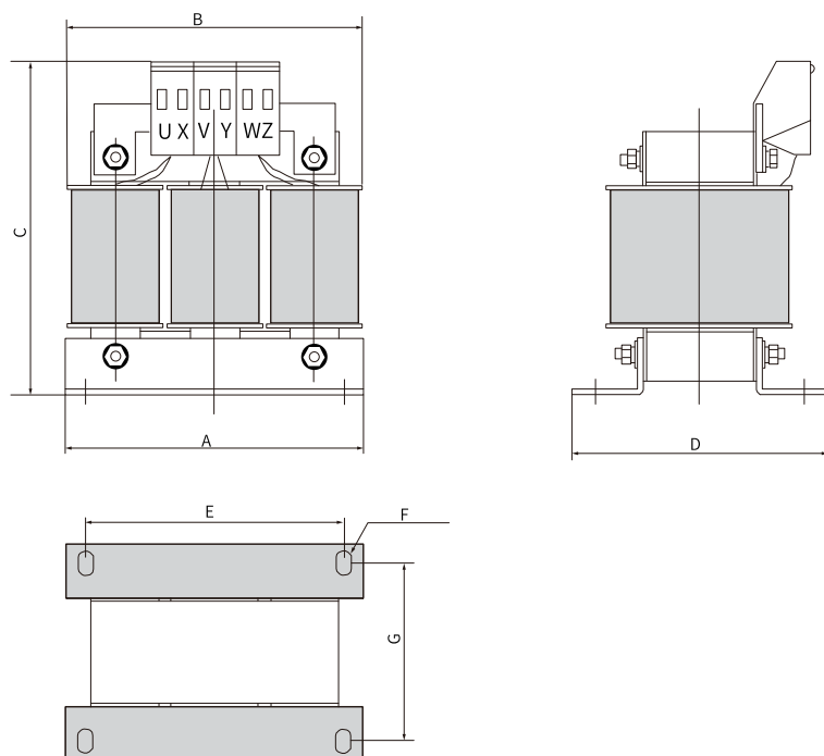
图7-9 5A-10A交流输出电抗器尺寸图
