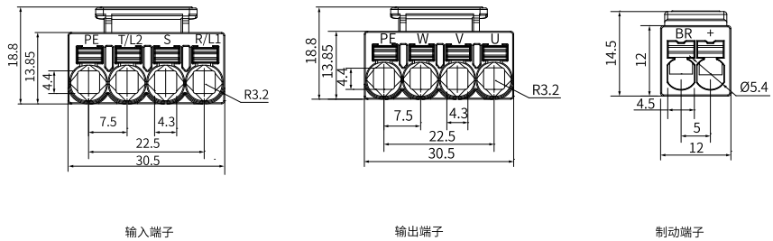
图9-20 T2机型主回路端子尺寸（单位：mm）
