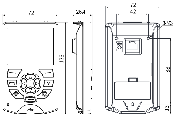
图7-1 SOP-20-810外引操作面板尺寸（单位：mm）
