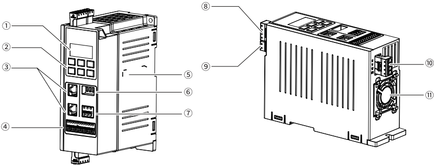
图2-1 产品部件示意图
