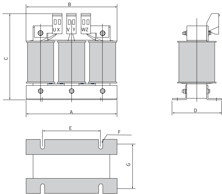
图7-10 15A交流输出电抗器尺寸图
