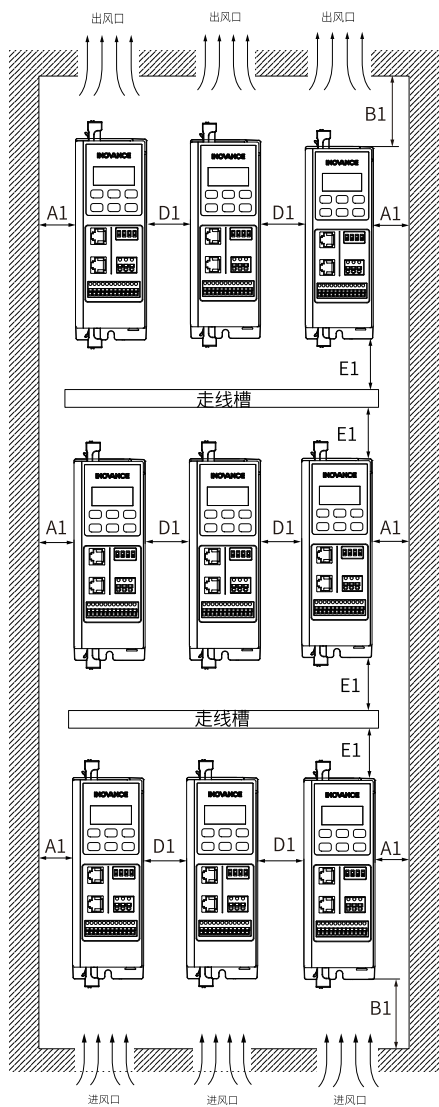
正视图
