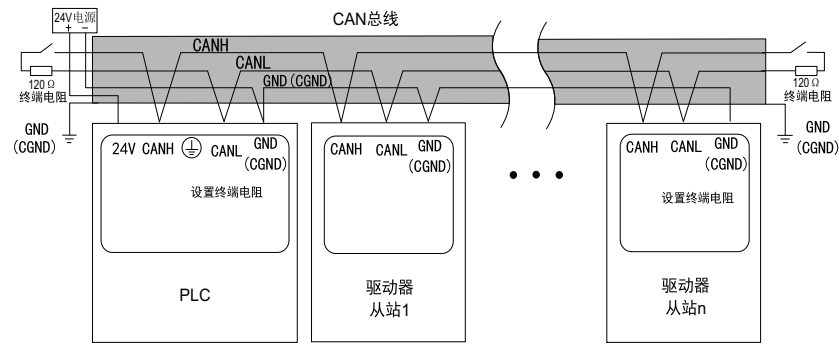
图9-5 CAN总线连接拓扑结构
