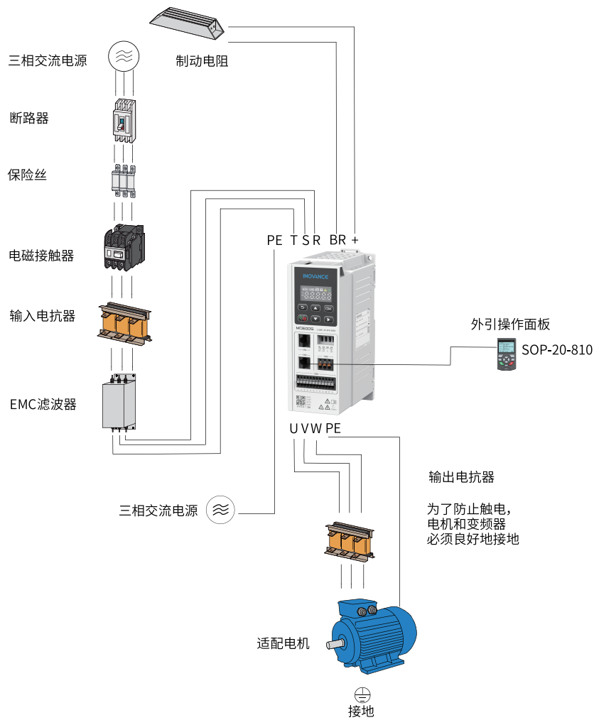
图9-15 系统连接图
