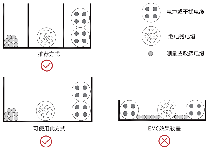
图9-13 多类电缆铺设方法示意图
