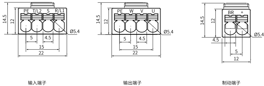
图9-19 T1机型主回路端子尺寸图（单位：mm）
