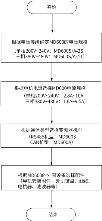
图4-1 选型流程图
