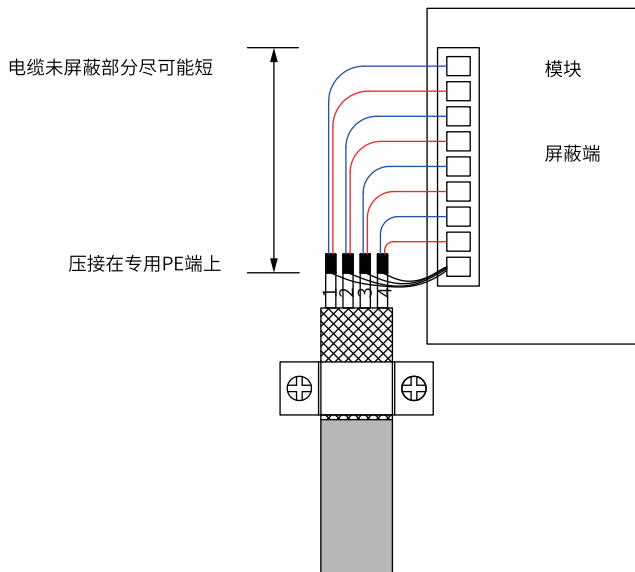
图9-14 屏蔽线处理要求示意图
