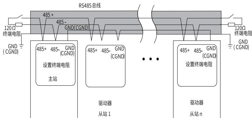
图9-6 RS485总线连接拓扑结构
