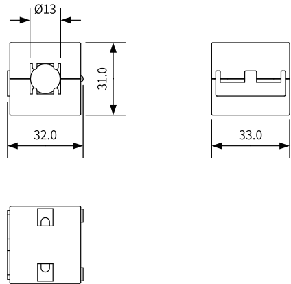
图7-15 磁扣尺寸图（单位：mm）
