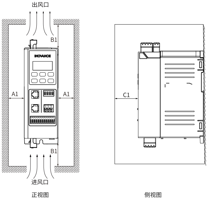
图8-1 安装空间示意图（单设备安装）
