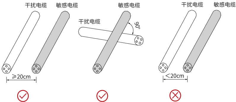
图9-8 干扰电缆与敏感电缆布线示意图
