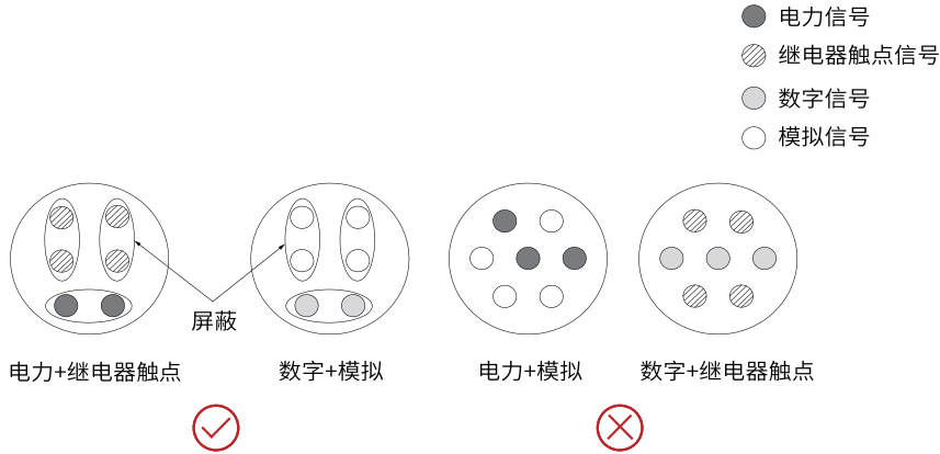
图9-10 多芯电缆布线示意图
