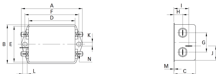
图7-12 FN2090系列滤波器尺寸图（单位：mm）
