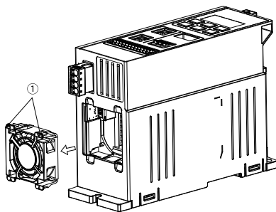
图8-6 风扇拆卸示意图
