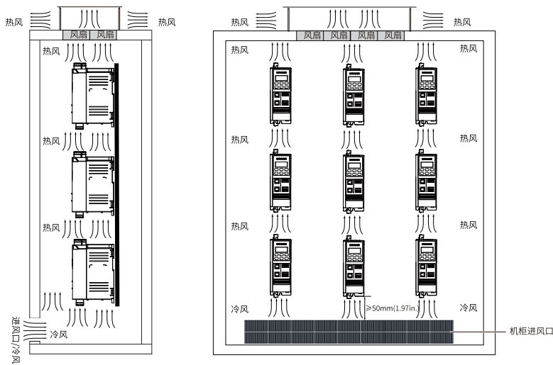
图8-5 机柜进风口开口位置示意图
