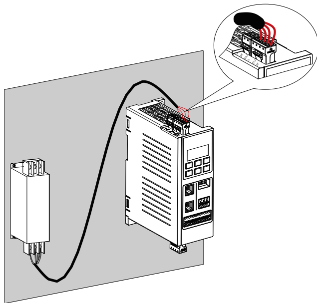
图9-1 EMC滤波器安装示意图
