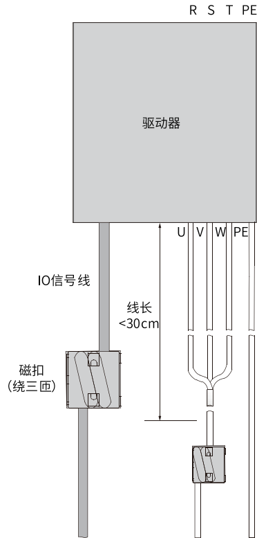
图9-3 磁扣安装示意图
